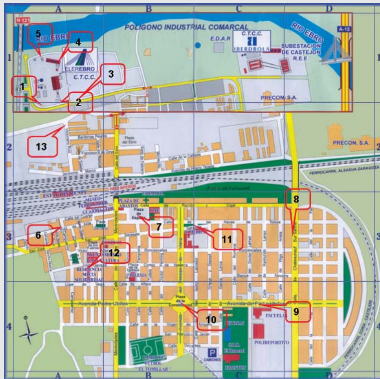
Puntos de medición de ruido
